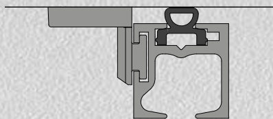
Montage met schaduwvoeg en pees
