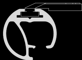
Plafondsteun met schaduwvoeg
