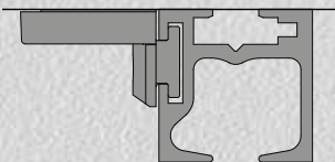
Montage direct aan het plafond
